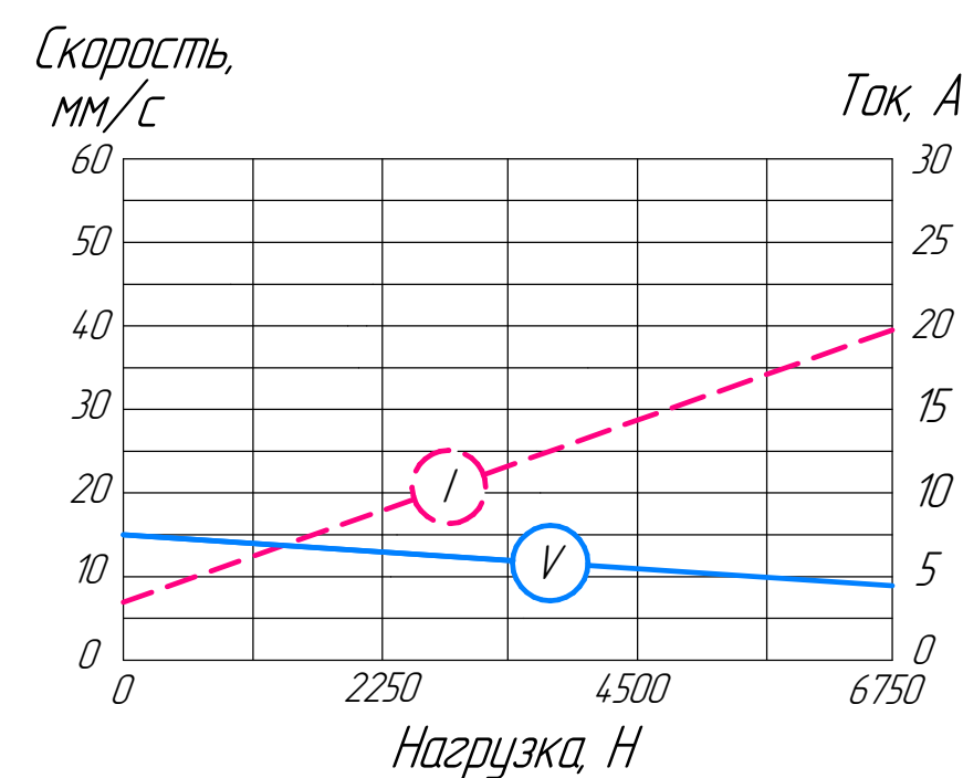
Графики зависимости скорости перемещения штока и тока потребления от осевой нагрузки при напряжении питания V=12 В и передаточном отношении редуктора i=20
