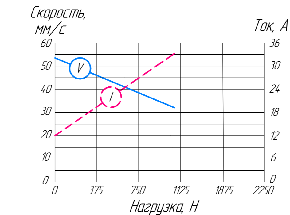
Графики зависимости скорости перемещения штока и тока потребления от осевой нагрузки при напряжении питания V=12 В и передаточном отношении редуктора i=5
