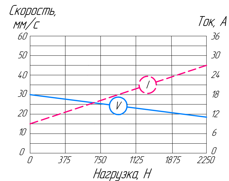
Графики зависимости скорости перемещения штока и тока потребления от осевой нагрузки при напряжении питания V=12 В и передаточном отношении редуктора i=10
