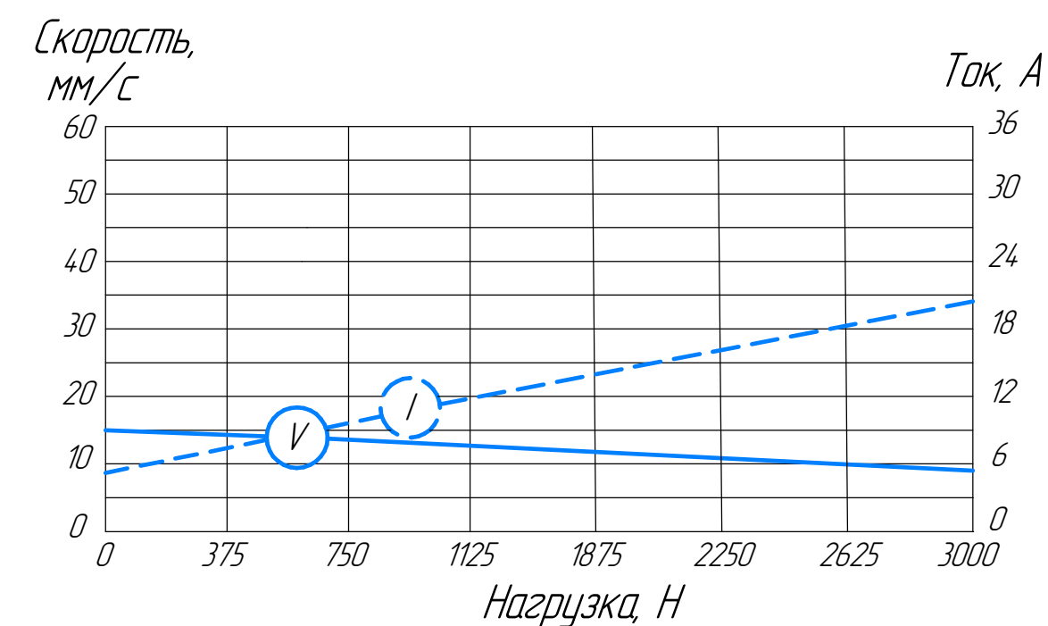
Графики зависимости скорости перемещения штока и тока потребления от осевой нагрузки при напряжении питания V=12 В и передаточном отношении редуктора i=20
