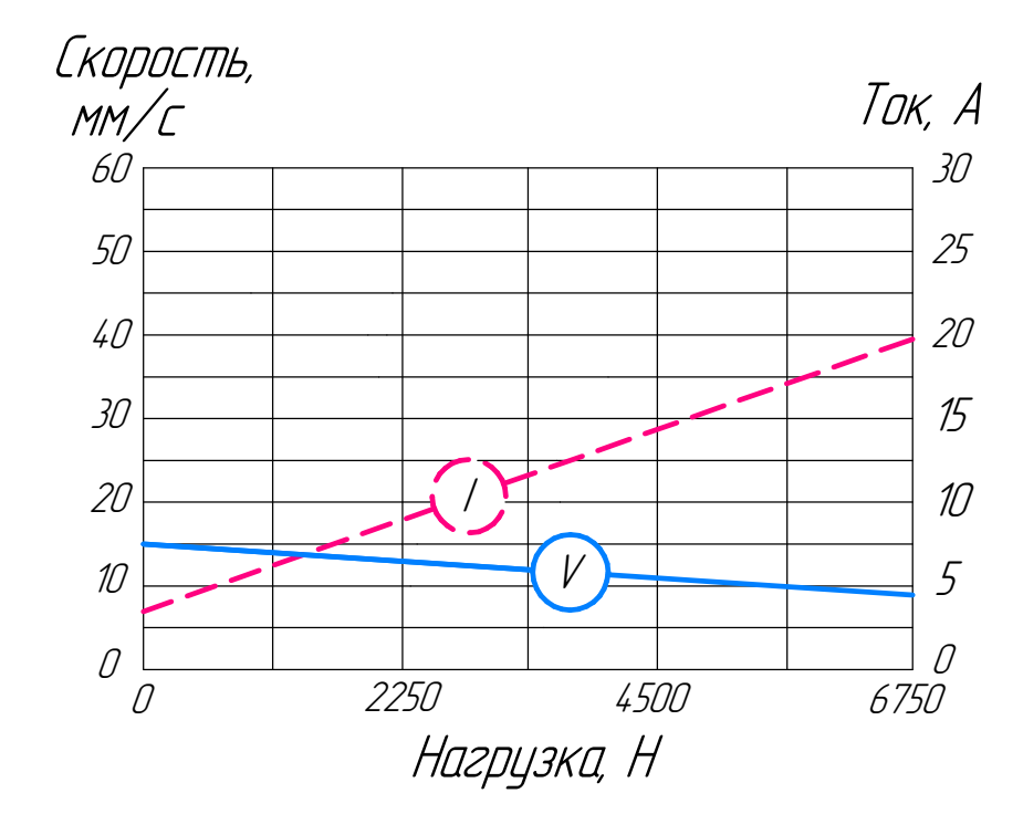
Графики зависимости скорости перемещения штока и тока потребления от осевой нагрузки при напряжении питания V=12 В и передаточном отношении редуктора i=20
