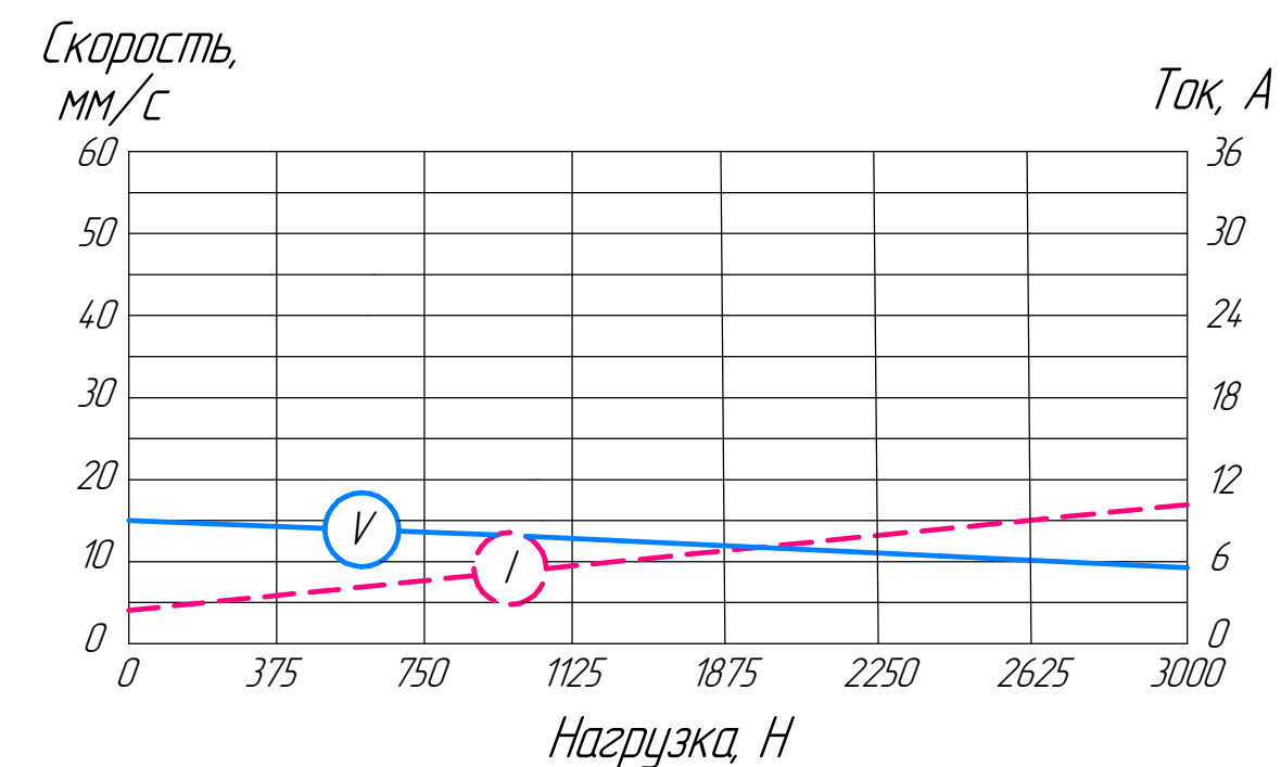
Графики зависимости скорости перемещения штока и тока потребления от осевой нагрузки при напряжении питания V=24 В и передаточном отношении редуктора i=20
